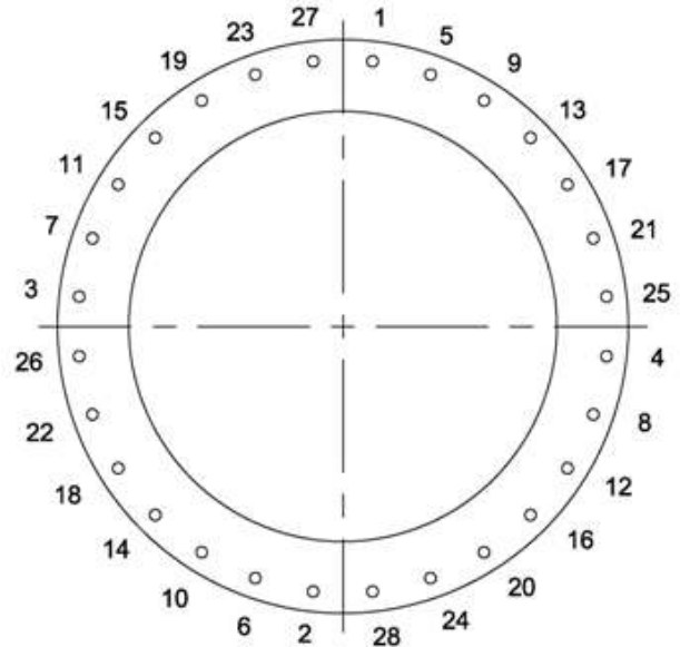
24" Side Manhole
