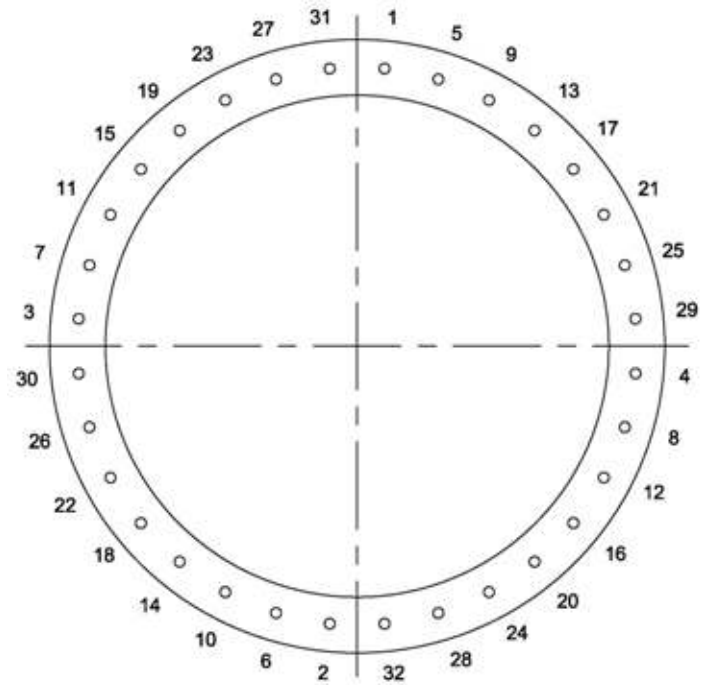
36" Side Manhole
